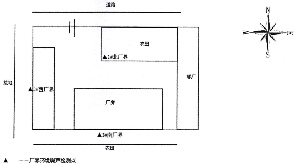
海燕接线盒有限公司 平面布局图与现场检测布点示意图
